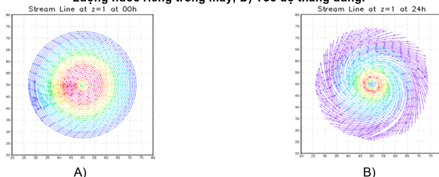
Hình 7. Trường đường dòng mực 1 (mức hội tụ) tại thời điểm ban đầu (A) và sau 24h tích phân(B)
