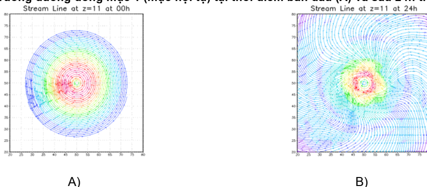
Hình 8. Trường đường dòng mực 11 (mức phân kì) tại thời điểm ban đầu (A) và sau 24h tích phân (B)
