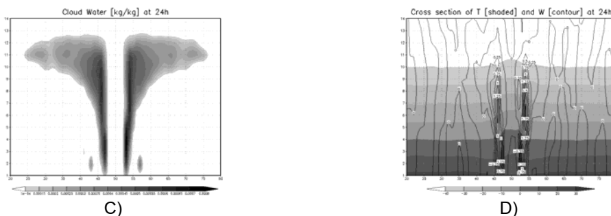
Hình 6. Sau 24 giờ tích phân của TH3: A) Trường độ ẩm riêng; B) Trường độ ẩm tương đối; C) Lượng nước riêng trong mây; D) Tốc độ thẳng đứng.
