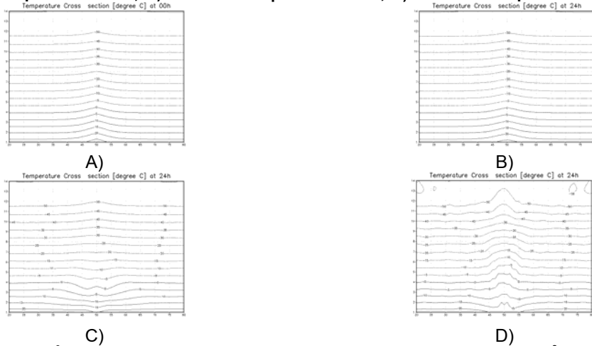
Hình 4. Mặt cắt thẳng đứng theo trục x qua tâm xoáy của nhiệt độ: A) Tại thời điểm ban đầu; B) Sau 24h tích phân của TH1; C) Sau 24h tích phân của TH2; D) Sau 24h tích phân của TH3
