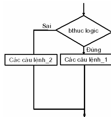
Hình 2.3 Cấu trúc IF dạng 3
