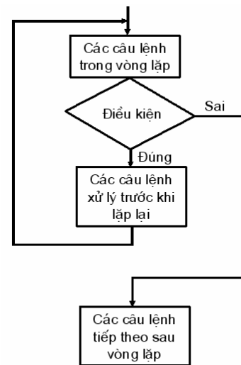
Hình 3.1 Cấu trúc lặp kết hợp IF và GOTO
