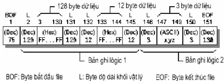
Hình 7.5 Cấu trúc file TEST3.TXT
