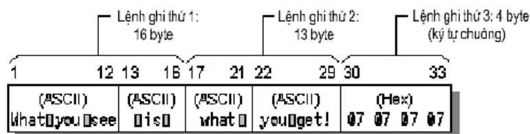
Hình 7.7 Cấu trúc file TEST5.TXT
