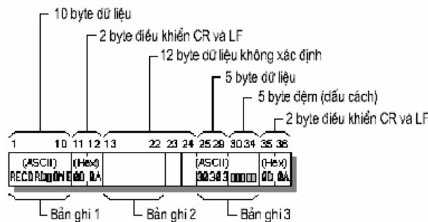
Hình 7.3 Cấu trúc file TEST2.TXT
