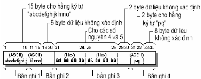
Hình 7.8 Cấu trúc file TEST6.TXT
