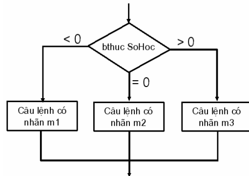
Hình 2.5 Cấu trúc IF số học
