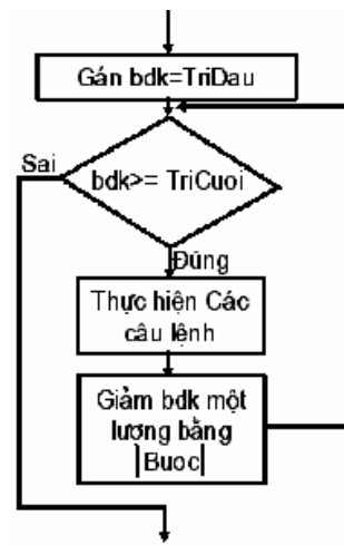
b) Trường hợp TriDau>=TriCuoi
