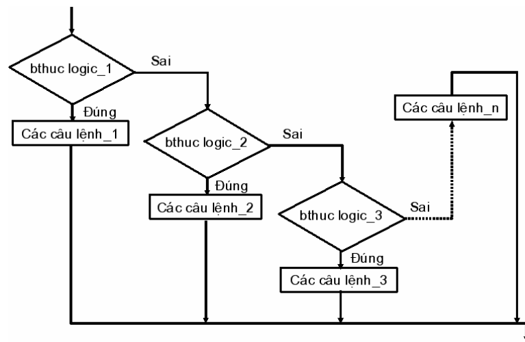
Hình 2.4 Cấu trúc IF dạng 4
