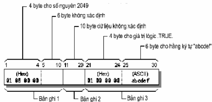
Hình 7.6 Cấu trúc file TEST4.TXT
